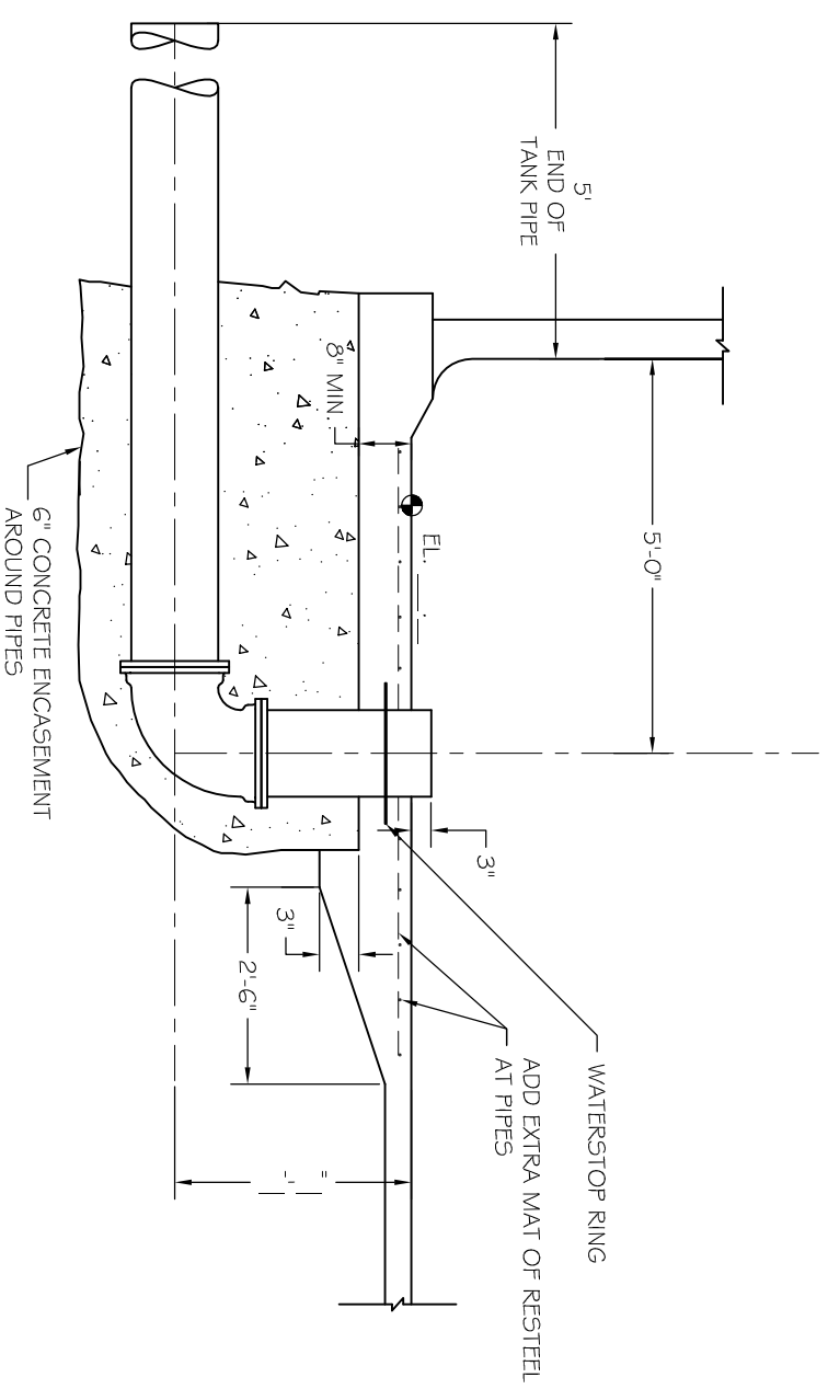
2" DIP INLET N.T.S
