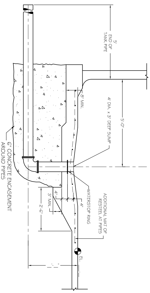
2" DIP DRAIN N.T.S
